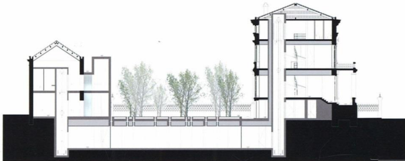
ALÇADO / CORTE CA03
