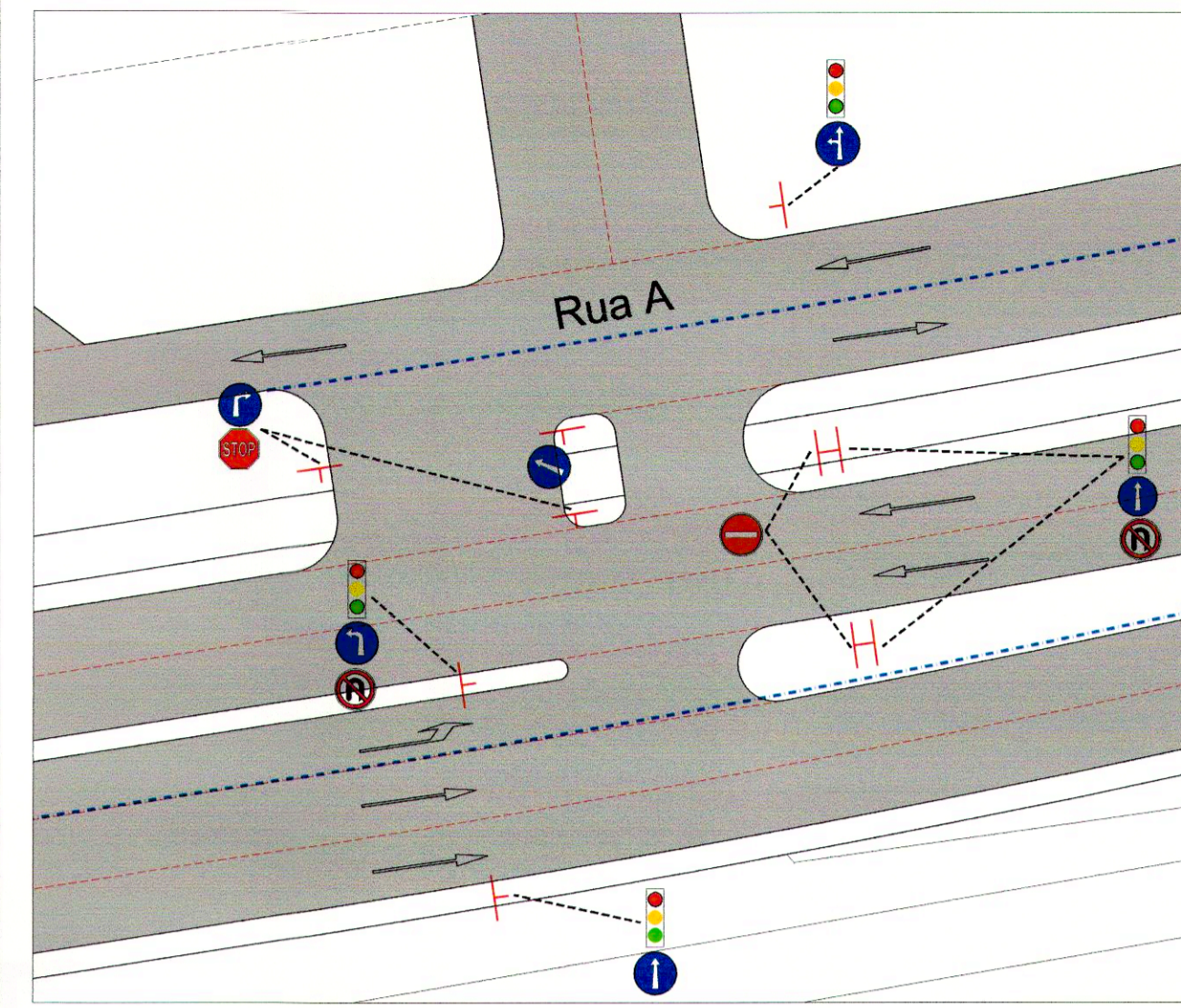
PORMENOR A - SINALIZAÇÃO (S/E)
