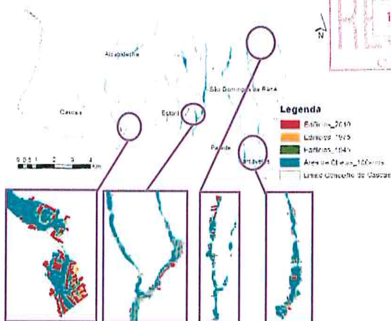
Figura 14 – Evolução da área edificada em zona de cheia com período de retorno de 100 anos.
