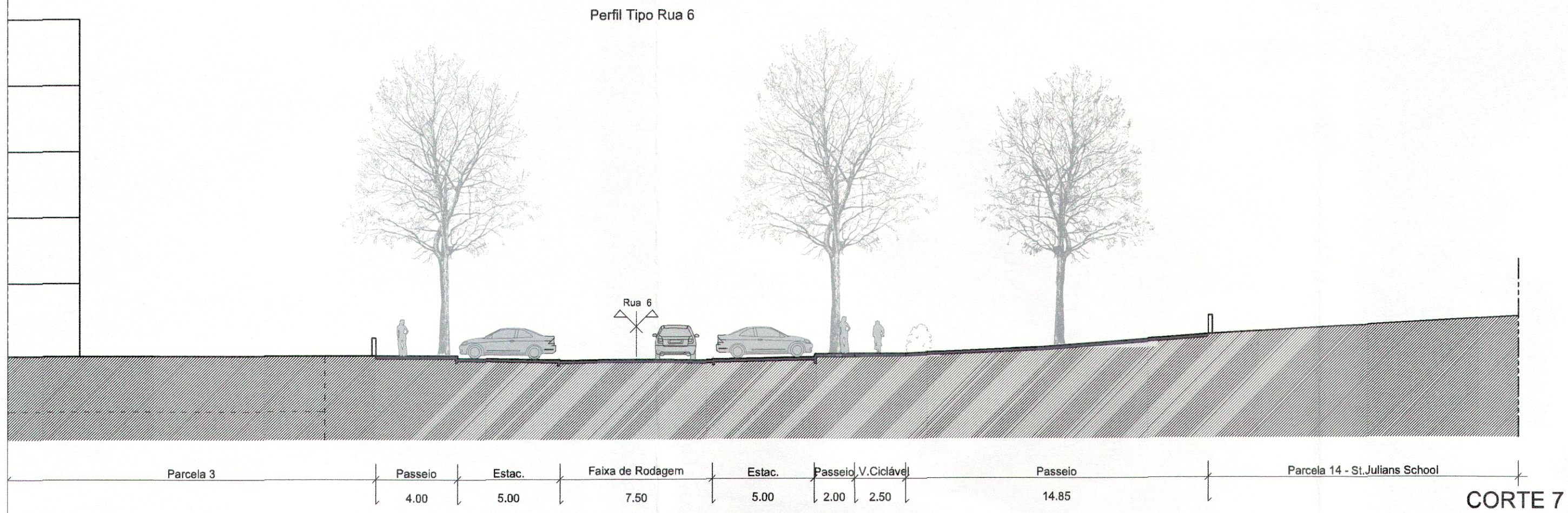
CORTE 7
