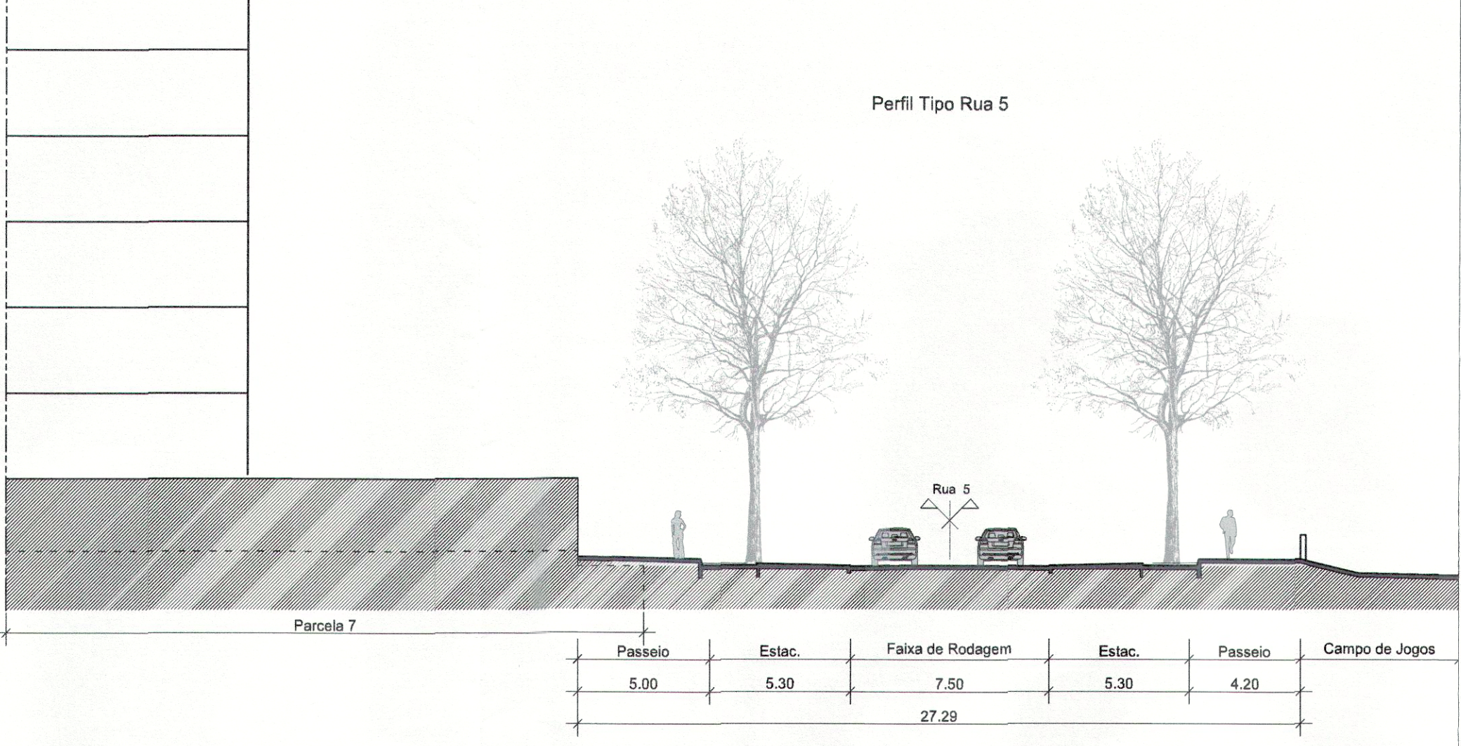
CORTE 11
