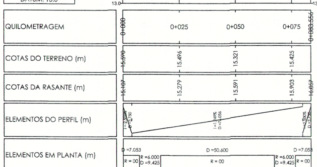
PERFIL RUA 7A KM TOTAL: 0+083.556 ESCALA HV: 1000/100 DATUM: 13.0
