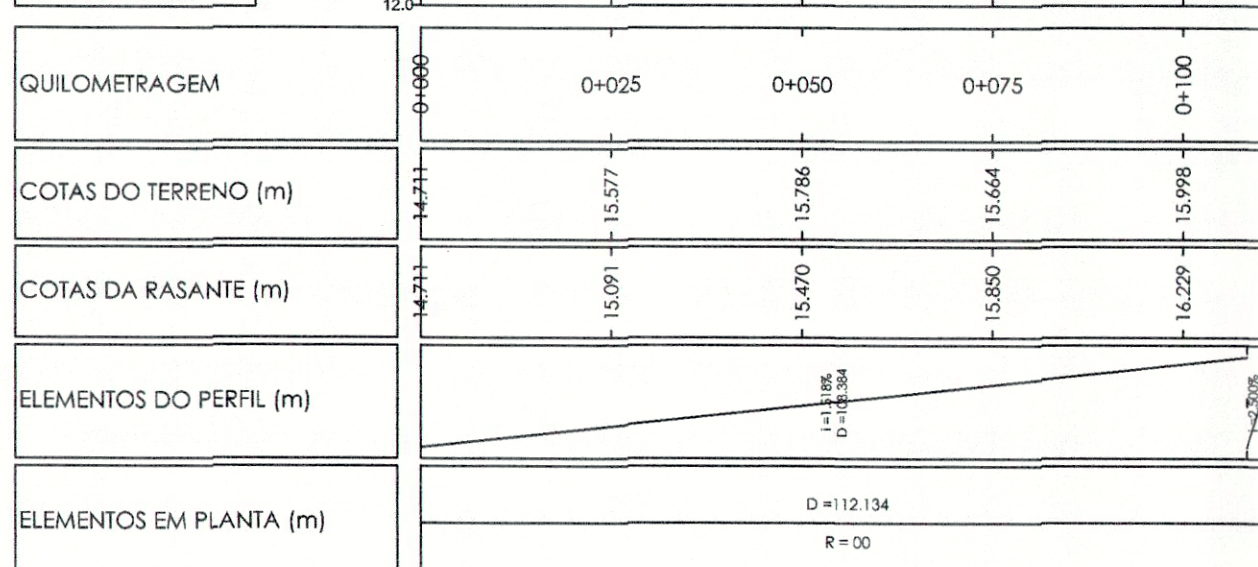
PERFIL RUA 7 KM TOTAL: 0+123.134 ESCALA HV: 1000/100 DATUM: 12.0
