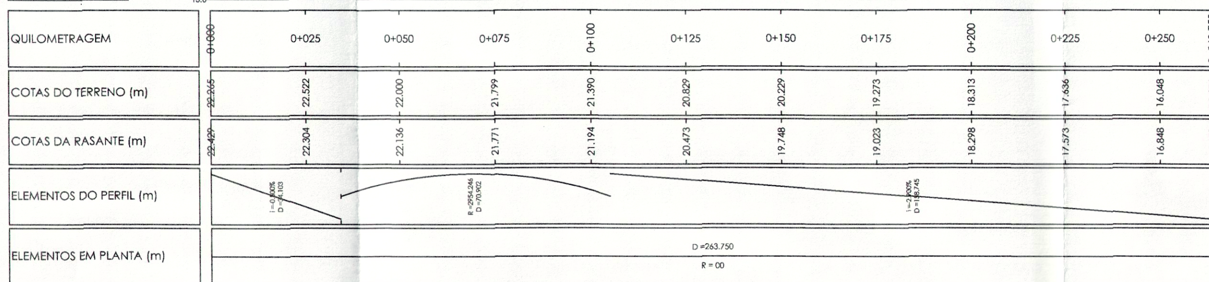
PERFIL RUA 2 KM TOTAL: 0+363.700 ESCALA HV: 1000/100 DATUM: 15.0
