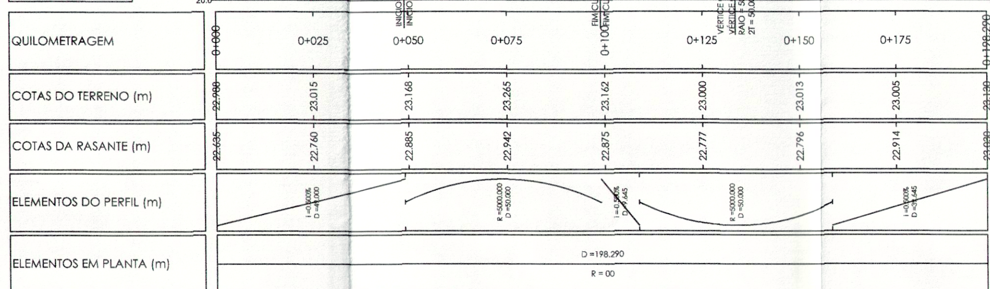
PERFIL RUA 1 KM TOTAL: 0+188.290 ESCALA HV: 1000/100 DATUM: 20.0
