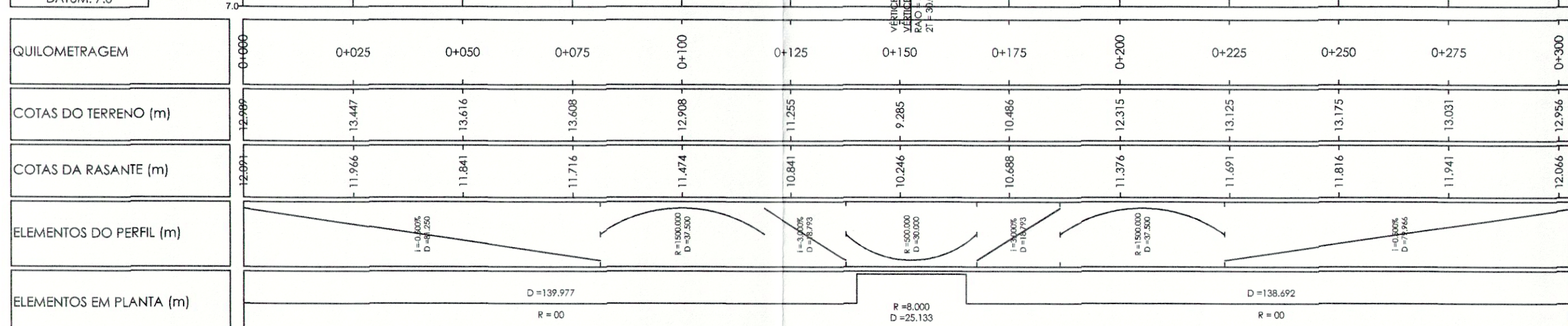
PERFIL RUA 8 KM TOTAL: 0+303.802 ESCALA HV: 1000/100 DATUM: 7.0
