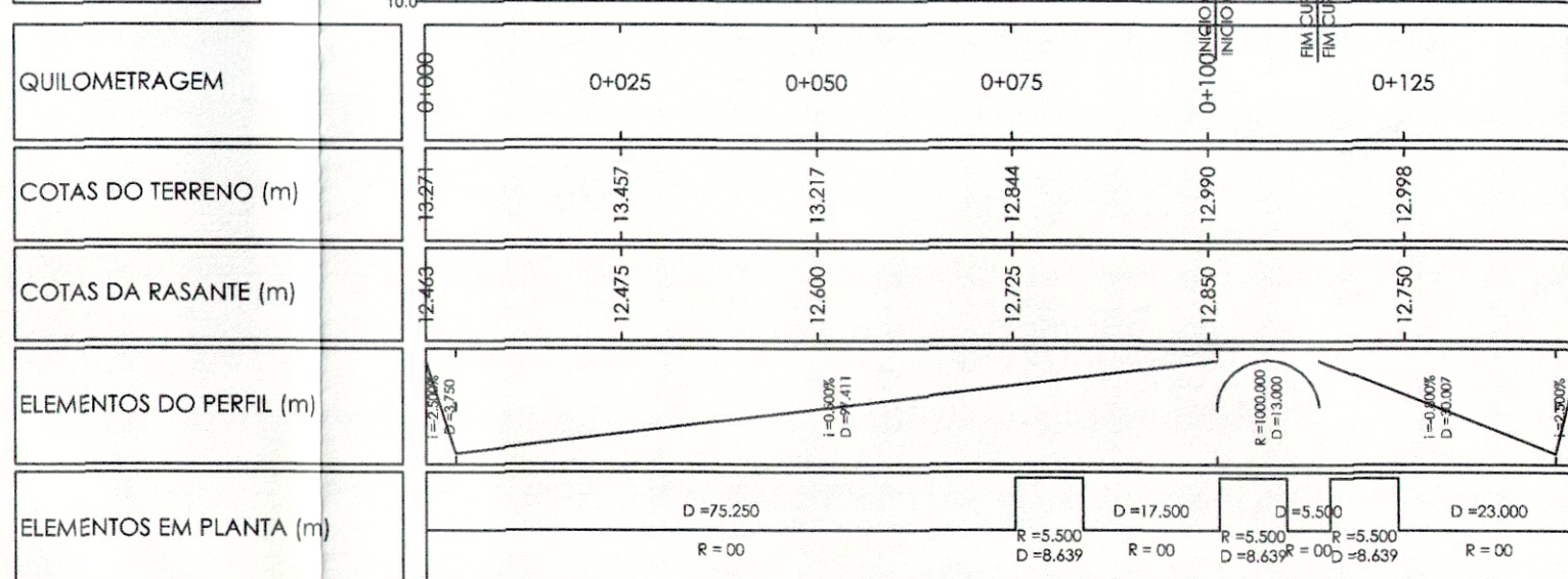
PERFIL RUA 3A KM TOTAL: 0+147.148 ESCALA HV: 1000/100 DATUM: 15.0
