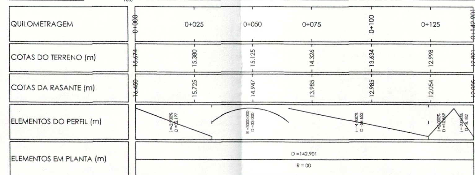
PERFIL RUA 3 KM TOTAL: 0+142.900 ESCALA HV: 1000/100 DATUM: 15.0
