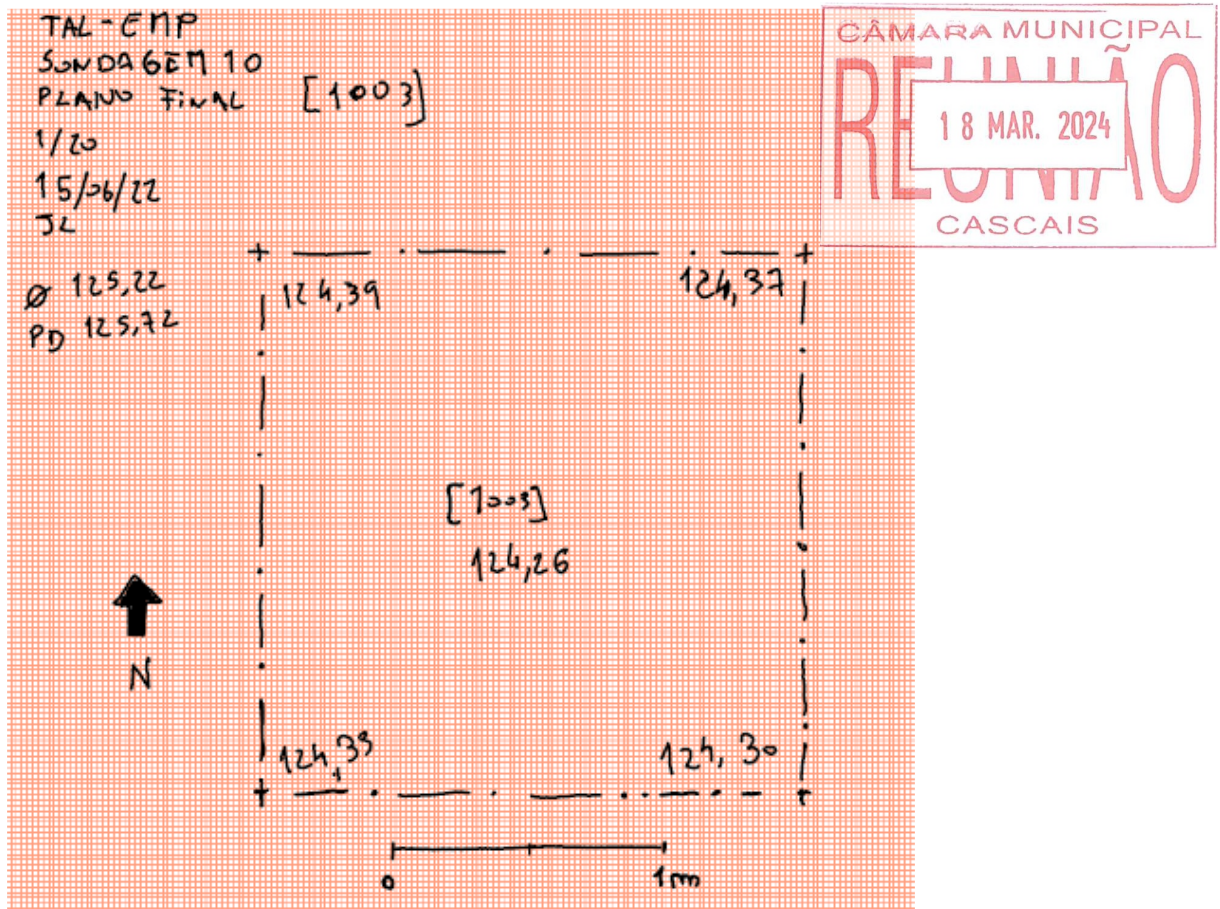
Desenho 19 - Plano final da sondagem 10 (escala 1:20).
