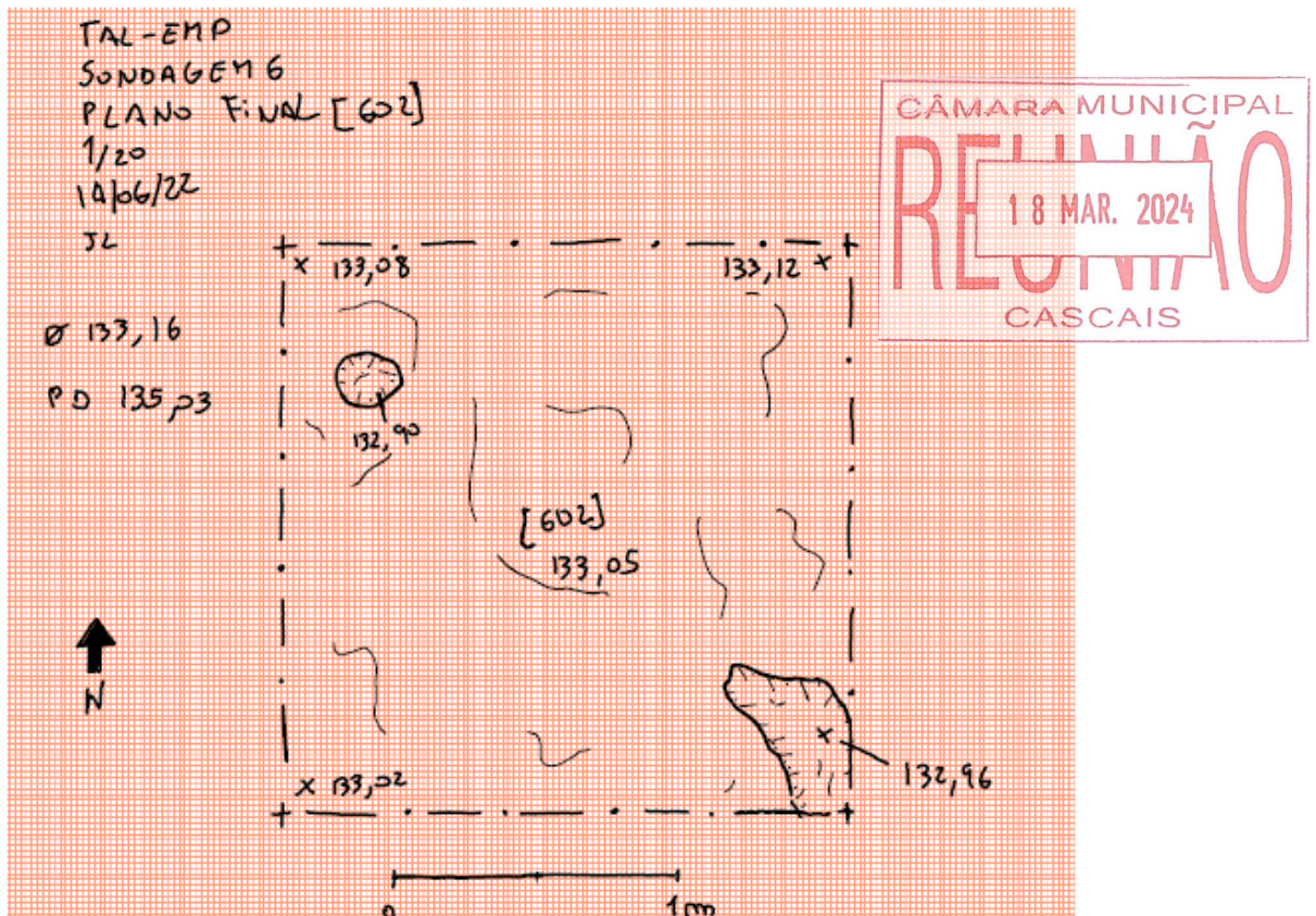
Desenho 11 - Plano final da sondagem 6 (escala 1:20).
