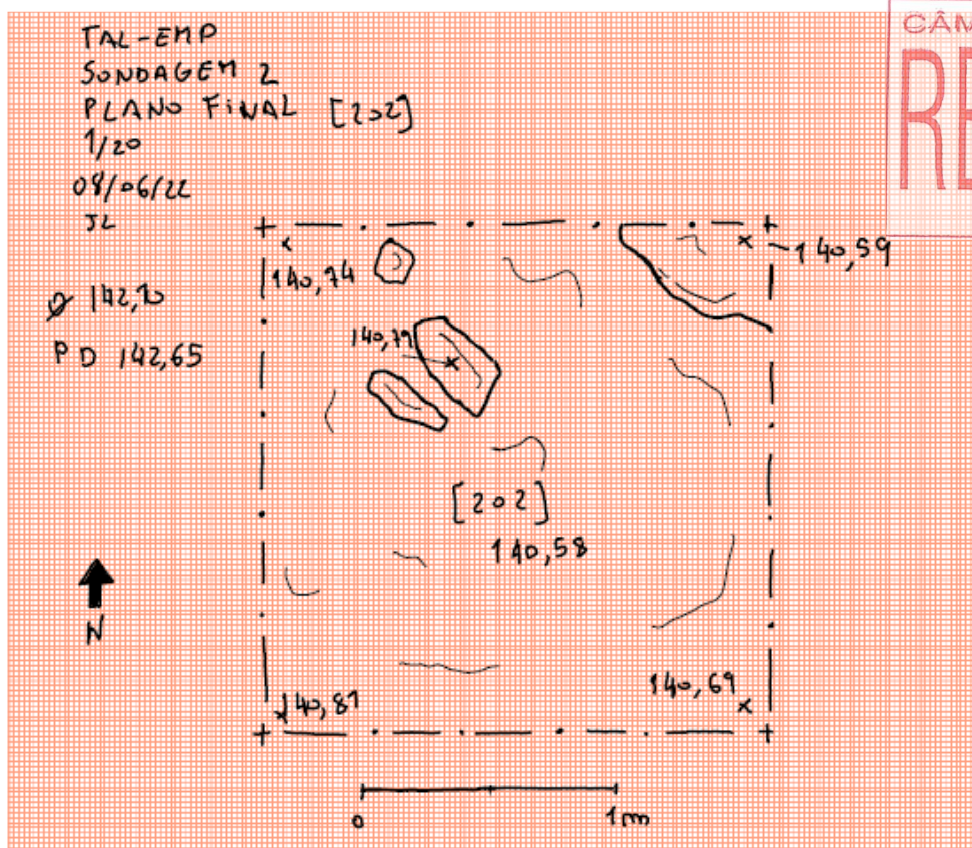
Desenho 3 - Plano final da sondagem 2 (escala 1:20).
