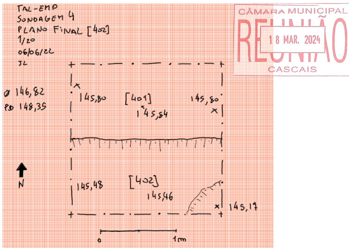
Desenho 7 - Plano final da sondagem 4 (escala 1:20).
