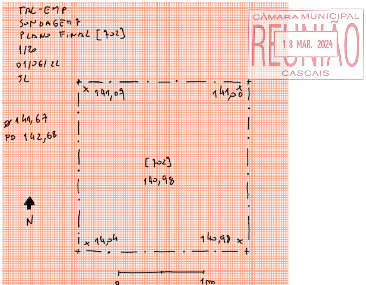
Desenho 13 - Plano final da sondagem 7 (escala 1:20).
