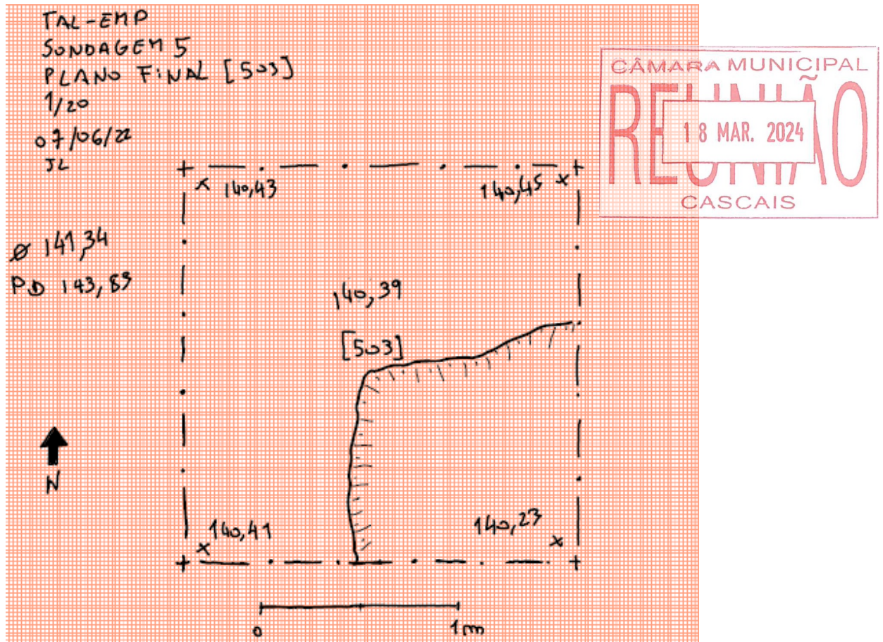
Desenho 9 - Plano final da sondagem 5 (escala 1:20).
