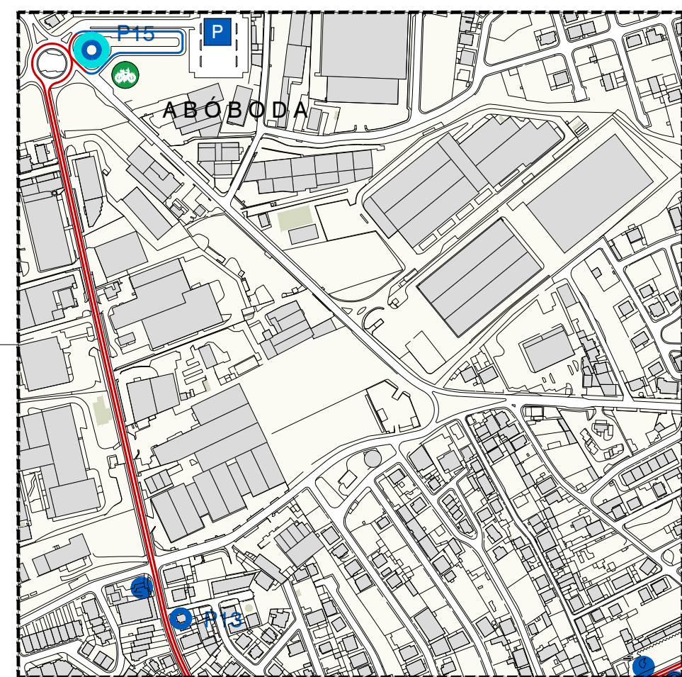
Proposta provisória para o traçado do corredor de TP Parede-Abóboda no troço junto à zona industrial da Abóboda
