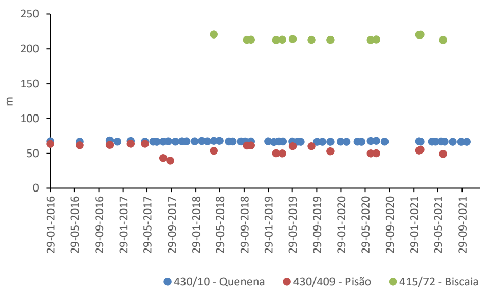
Figura 7 – Nível piezométrico nos pontos de água 430/10, 430/409 e 415/72
